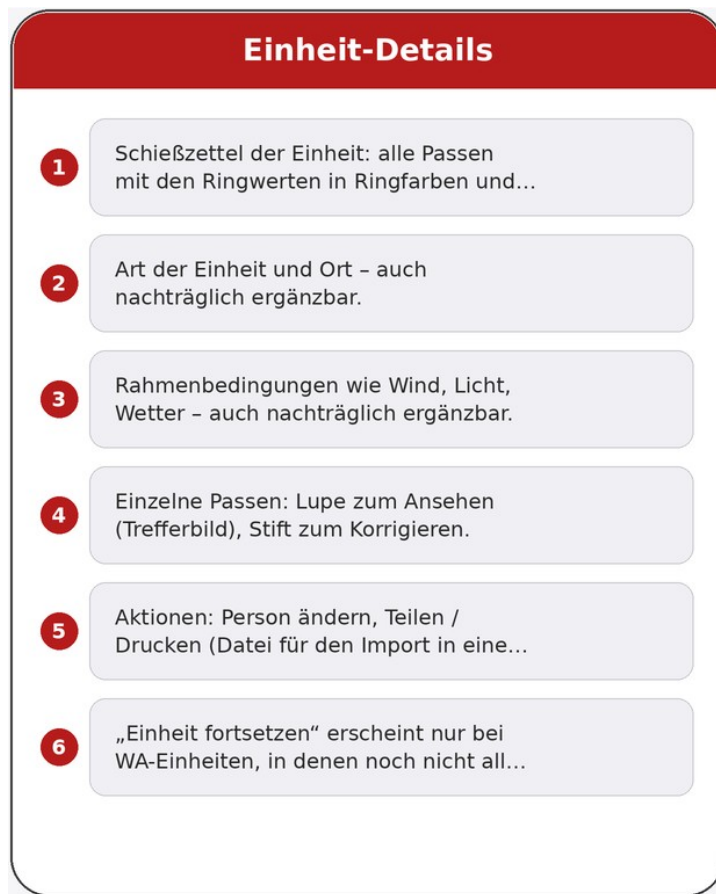
Abbildung 19: Einheit-Details
