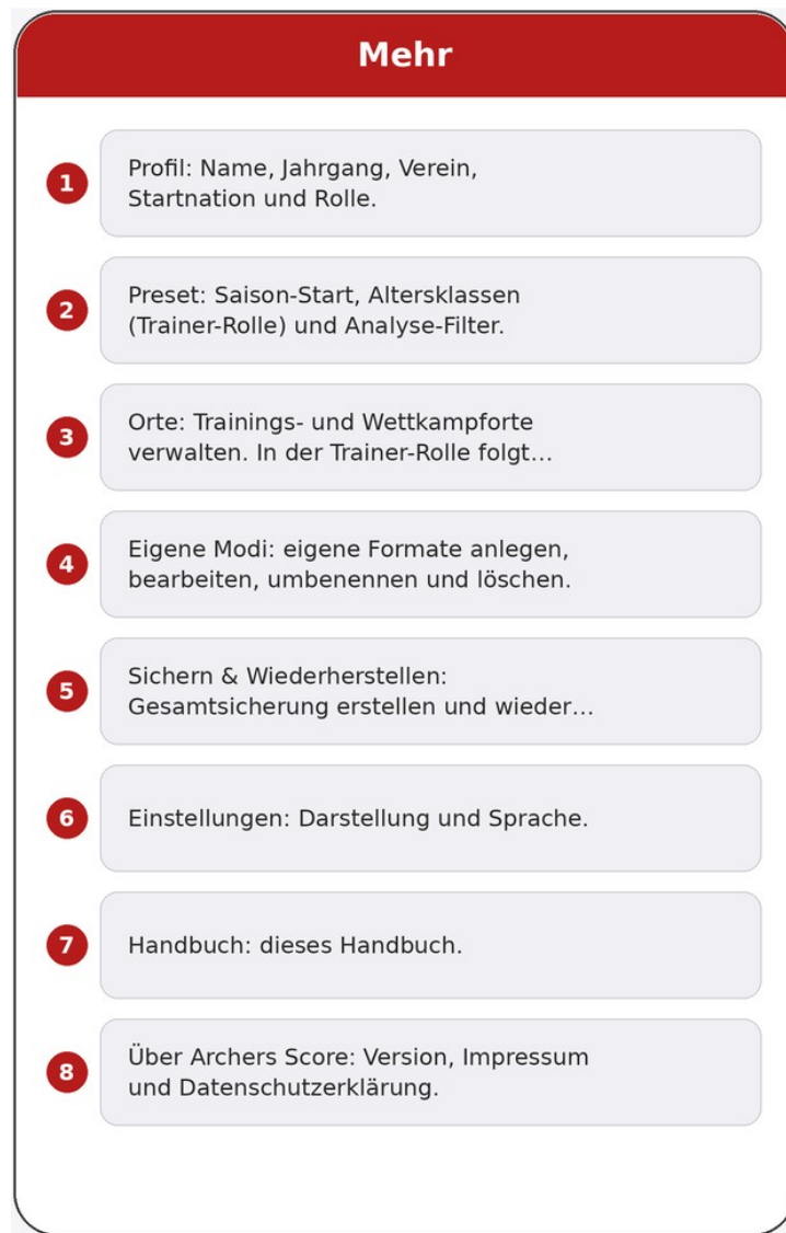
Abbildung 23: Mehr
