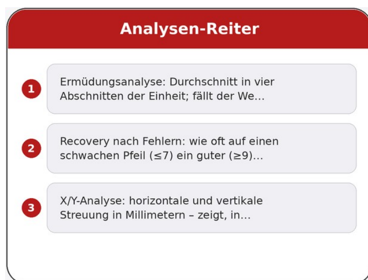
Abbildung 22: Analysen-Reiter
