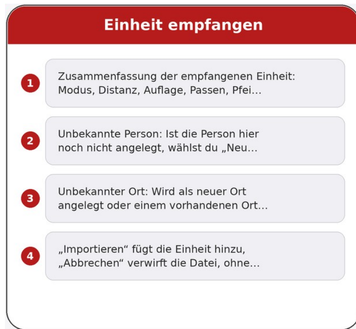
Abbildung 29: Einheit empfangen
