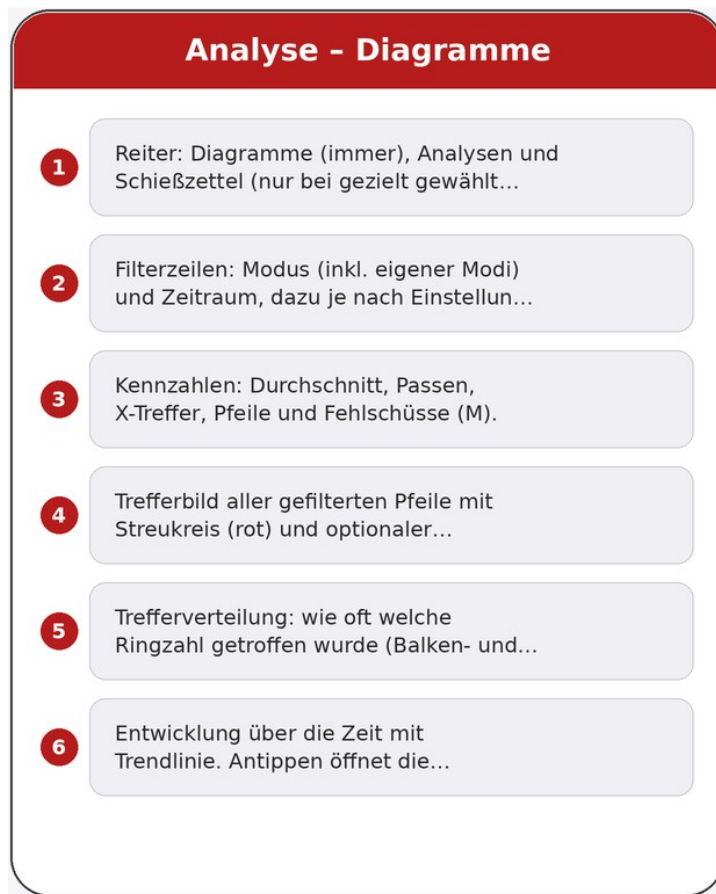
Abbildung 20: Analyse - Diagramme
